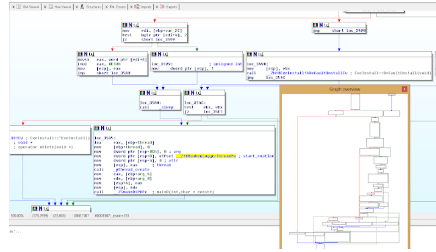
Keylogger function
